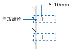
图3 固定螺栓
